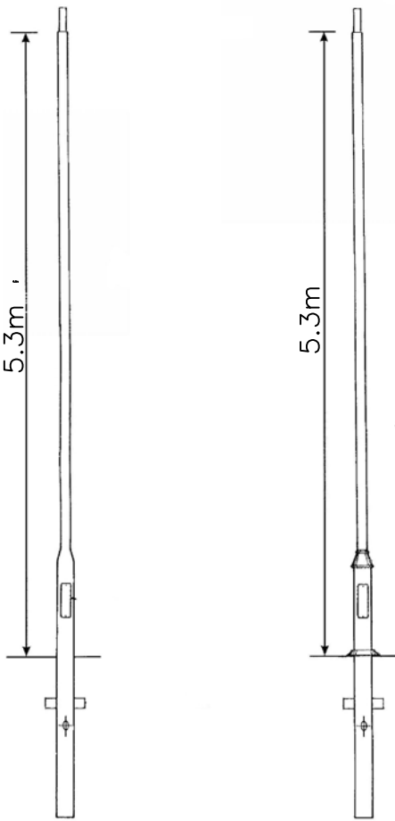
Avon Column
